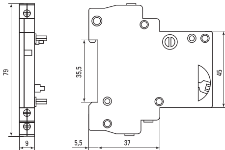
Рис. 2 Габаритный и установочный размеры АК
