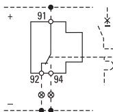
Рис. 1 Схема подключения
