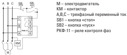
Рис. 4 Схема подключения реле
