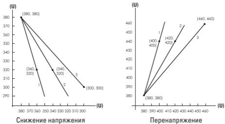
Рис.1 Рабочие характеристики перенапряжения/снижения напряжения
