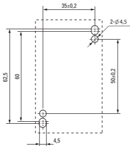
Рис. 3 Установочные размеры на монтажную панель
