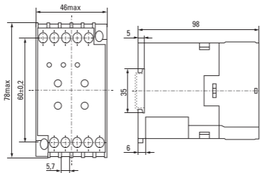
Рис. 2 Габаритные размеры РКФ-11.
