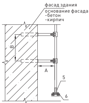
Рис. 2 - Узел крепления молниеприёмника к стене
