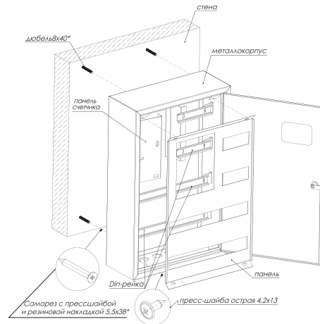
Рис.1. Схема монтажа
