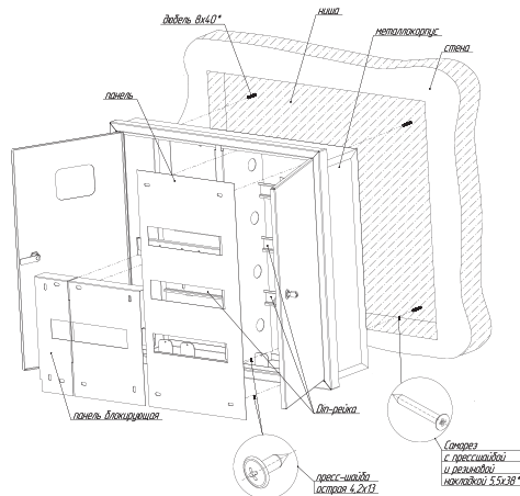
Рис.1. Схема монтажа
