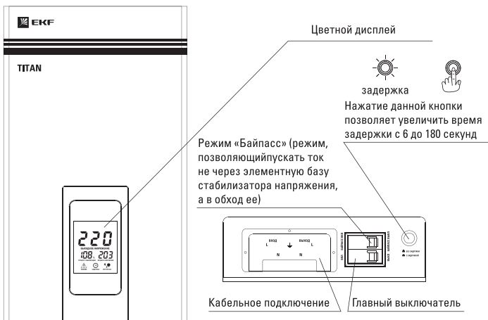
Рис. 3 Внешний вид стабилизатора W-3000-5000
