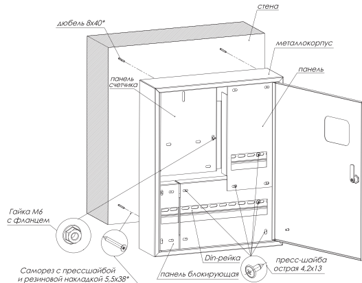
Рис.1. Схема монтажа
