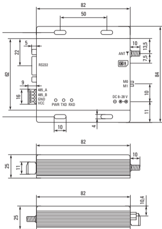
Рисунок 2-а – Габаритные и установочные размеры модема
