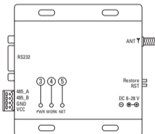
Рисунок 1-а – Внешние элементы модема
