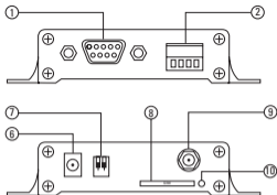
Рисунок 1-б – Внешние элементы модема
