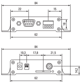
Рисунок 2-6 – Габаритные и установочные размеры модема
