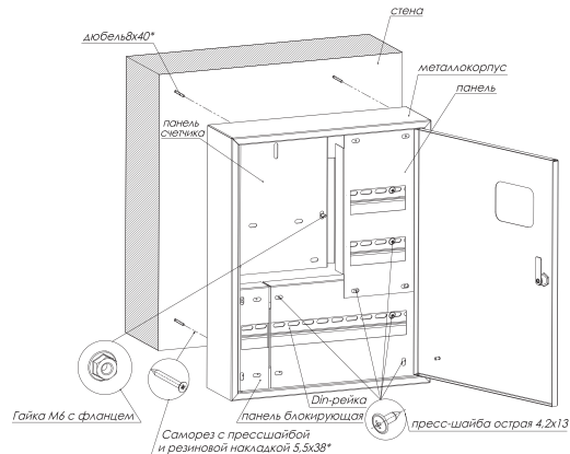
Рис.1. Схема монтажа
