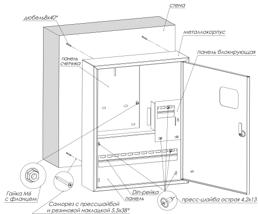
Рис.1. Схема монтажа
