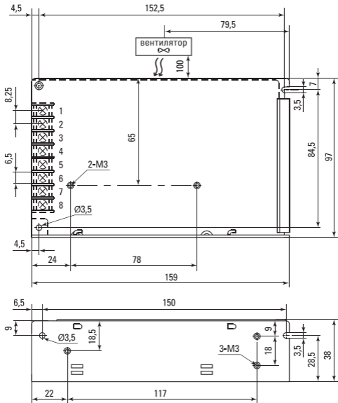
Рис 1. Габаритные размеры MPSu-55W-24
