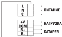
Рис 3. Схема подключения
