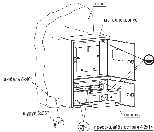
Рис.1. Схема монтажа
