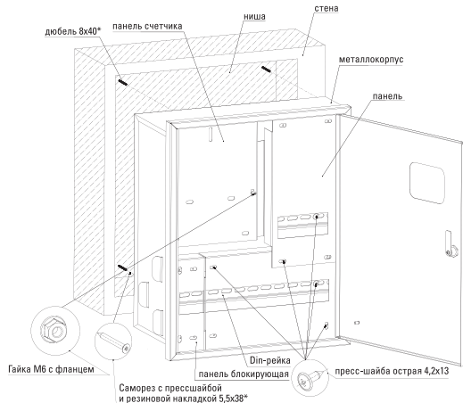
Рис.1. Схема монтажа
