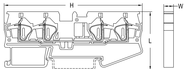
JXB-ST - 4 вывода
