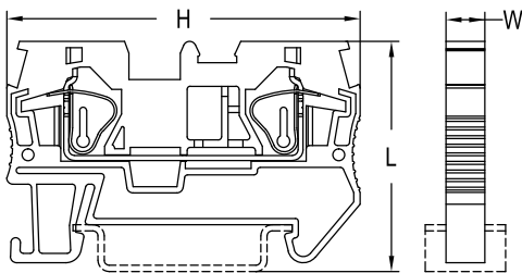
JXB-ST - двойная
