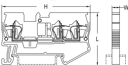
JXB-ST - 3 вывода
