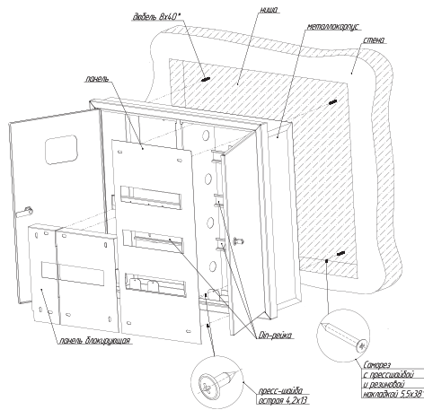
Рис.1. Схема монтажа
