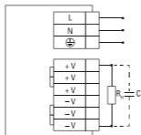
Рис 8. Схема подключения (MPS-200W-24, MPS-350W-24)
