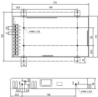
Рис 5. Габаритные размеры (MPS-200W-24, MPS-350W-24)
