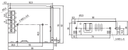
Рис 1. Габаритные размеры (MPS-35W-24, MPS-50W-24)
