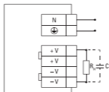
Рис 7. Схема подключения (MPS-100W-24, MPS-150W-24)
